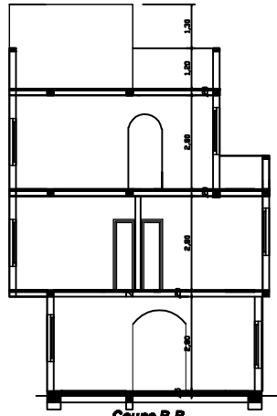
Coupe B-B
