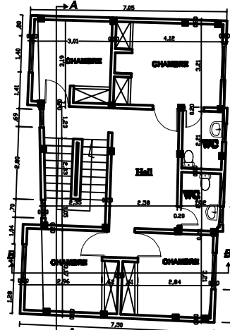
1 ER Etage
