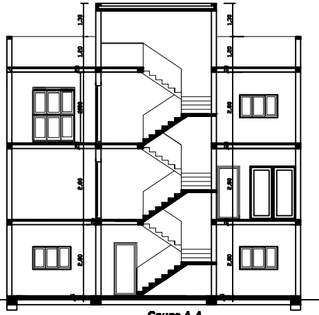
Coupe A-A
