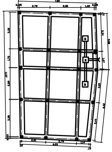
Fondations
